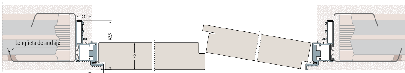
Marco en la pared de placa de yeso - Espesor pared acabada 100 mm
