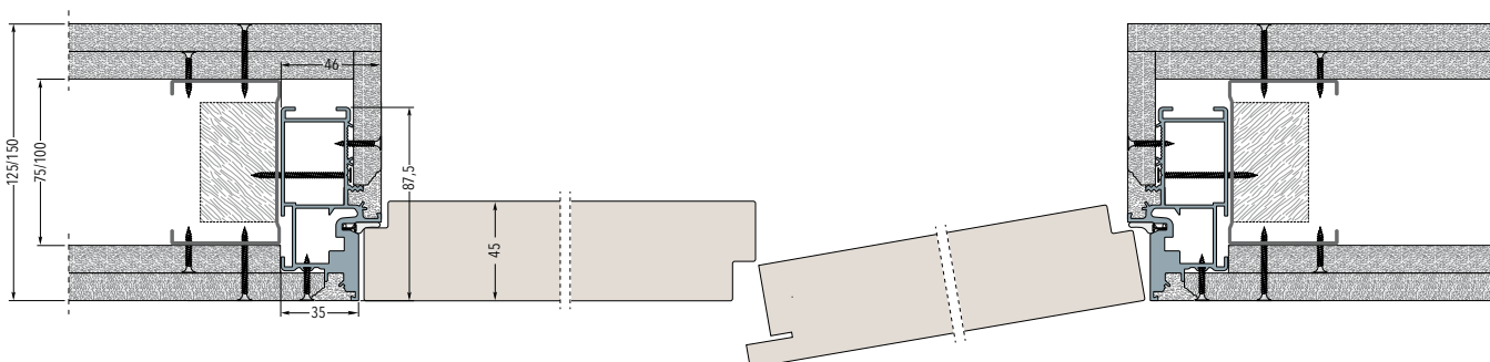
Marco en la pared de placa de yeso con dos placas - Espesor pared acabada 125/150 mm
