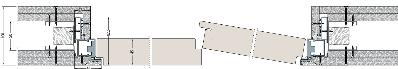
Marco en la pared de placa de yeso con dos placas - Espesor pared acabada 100 mm
