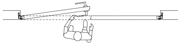
PUERTA IZQUIERDA TIRAR - PUERTA DERECHA FIJA
