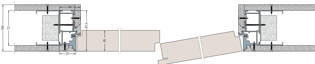
Marco en la pared de placa de yeso con dos placas - Espesor pared acabada 100 mm
